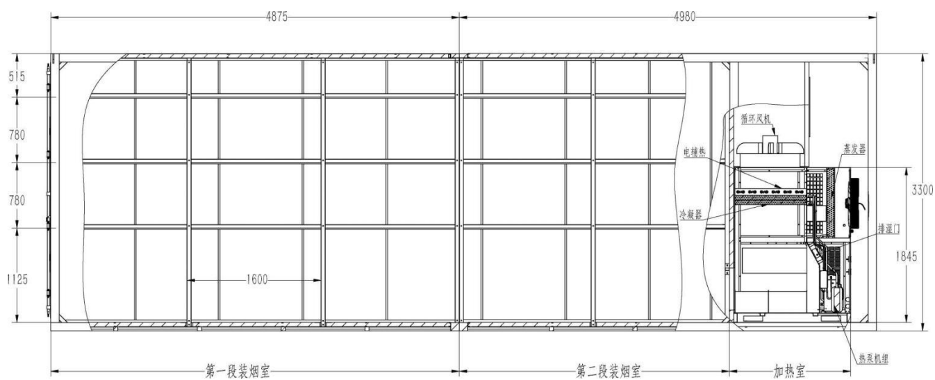
图 1 移动烤房整体结构图
