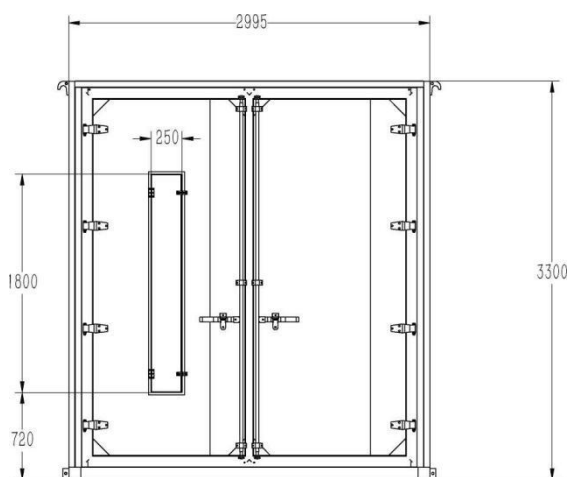
图 2 移动烤房后侧视图
