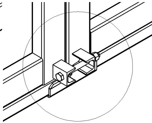
图 6 移动烤房下连接视图
