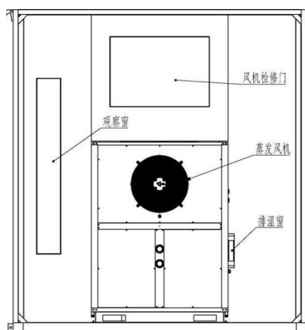
图 4 移动烤房左侧视图
