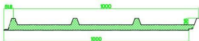
图 5 屋面板视图
