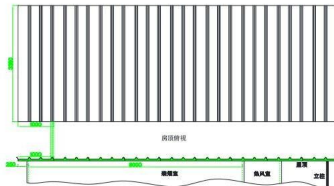
图 6 屋面板拼接
