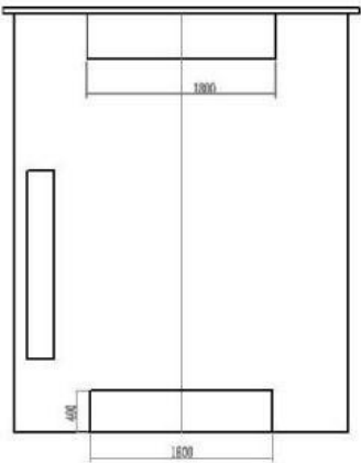
图 13 全部拆除后隔热墙视图
