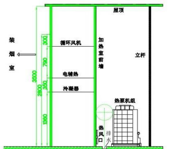
图 10 加热室内部结构图
