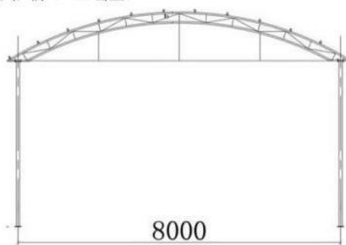
图 12 10 座连片烤房编烟棚示意图
