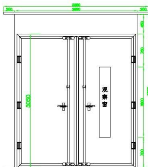
图 9 装烟室大门图
