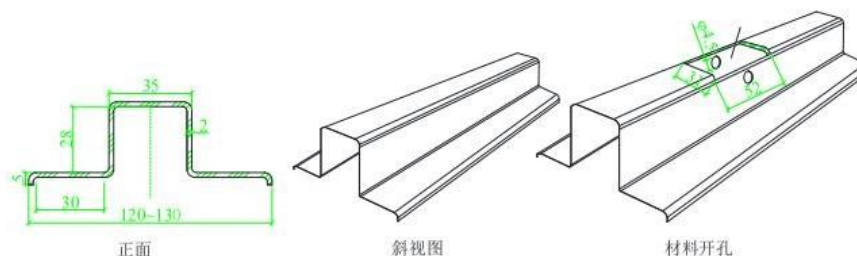
图 7 烟梁结构图
