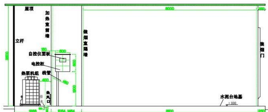
图 2 烤房右侧视图
