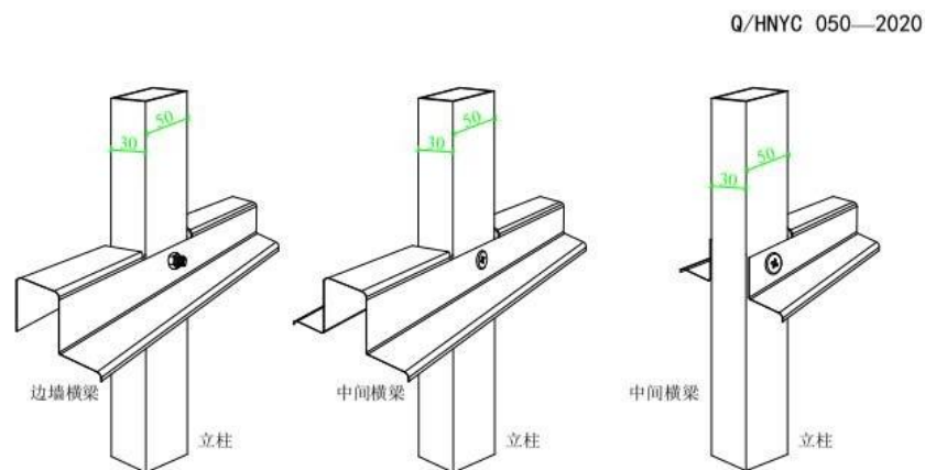
图 8 立柱与烟梁连接图
