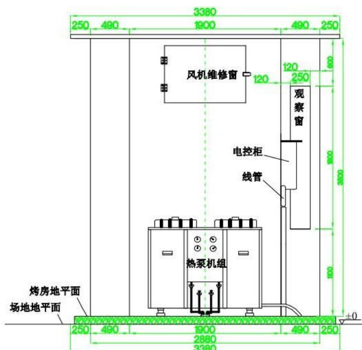
图 3 烤房前视图
