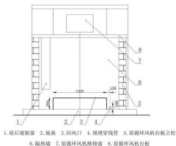
图 15 部分拆除后隔热墙视图
