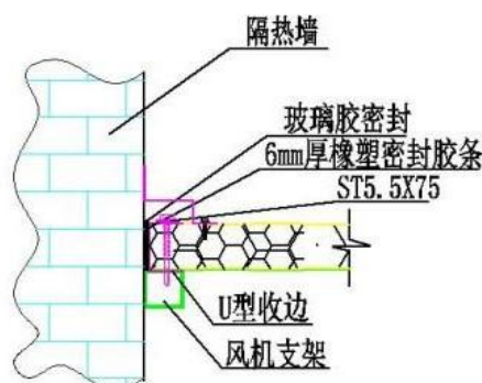
图 14 加热室与装烟室接缝处理
