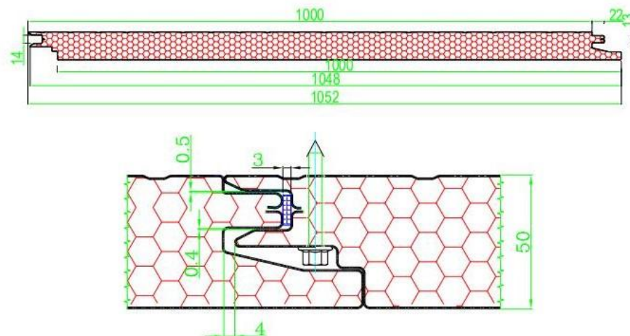
图 4 墙板及连接图
